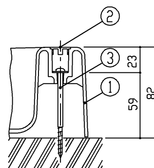
固定部詳細(1/3)
